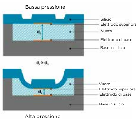
Sezione del sensore BAROCAP
